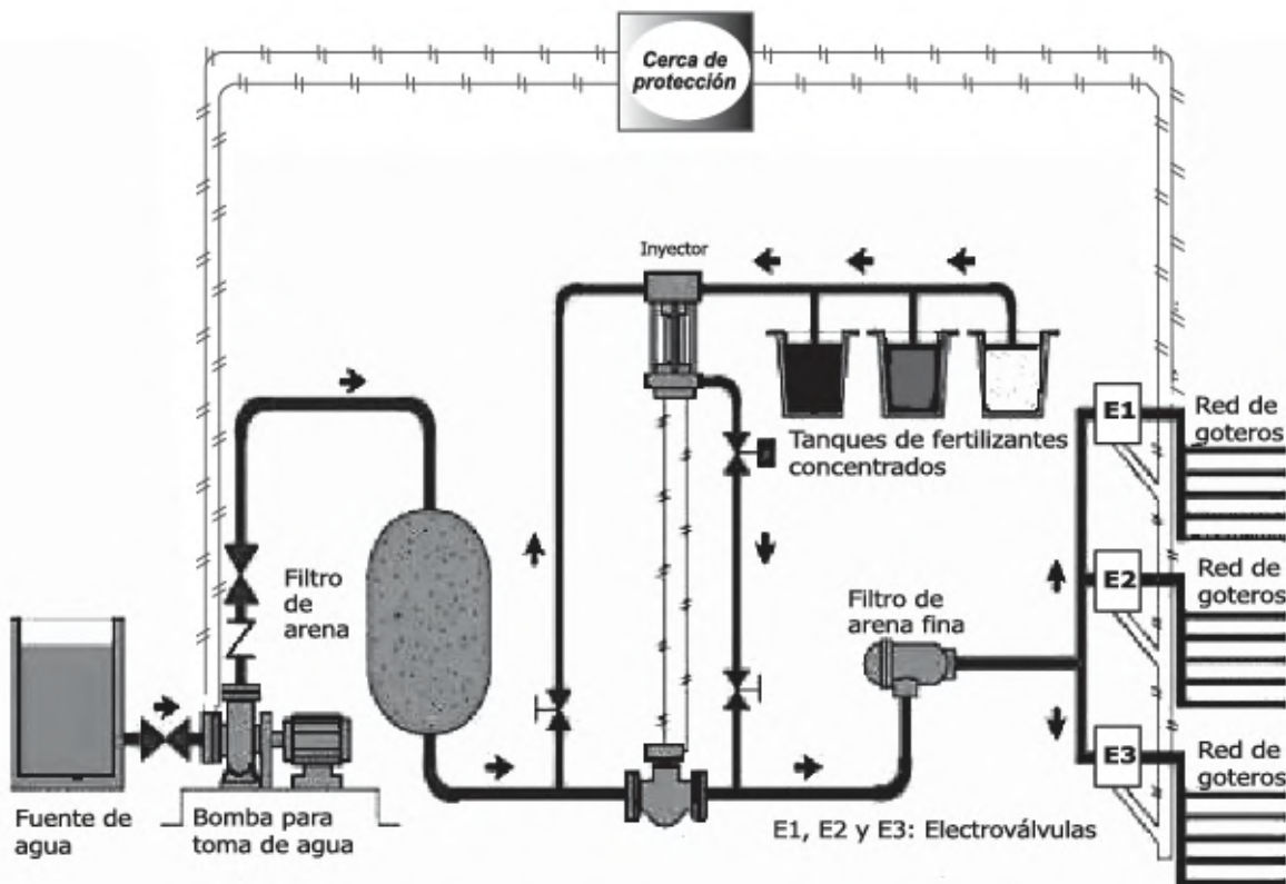
Figura 25. Esquema de un sistema de fertirrigación en café.
